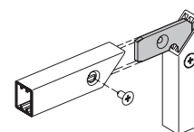
Montageset 70.103
