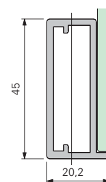
Profil GFR 45
