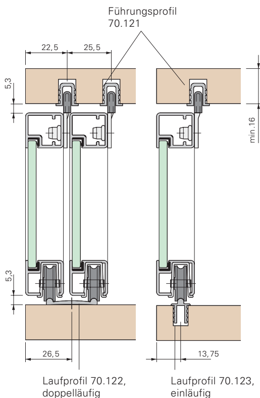
Beschlagset 70.119
