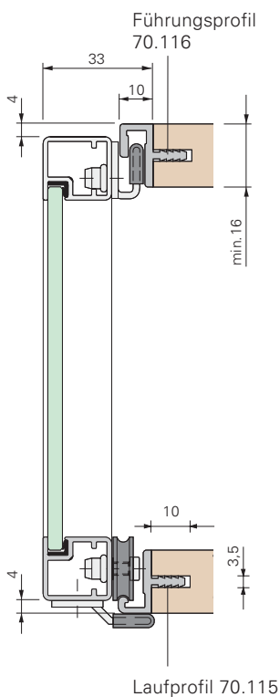
Beschlagset 70.113
