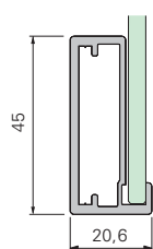
Profil SD 45
