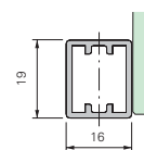
Profil GFR 19
