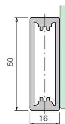
Profil GFR 50
