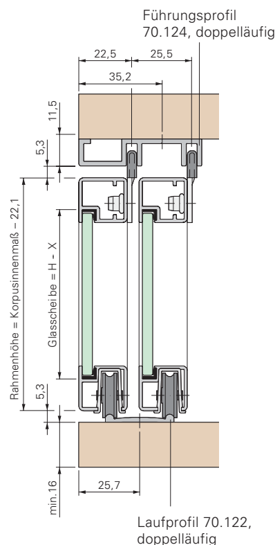
Beschlagset 70.119
