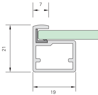
Profil DD7
