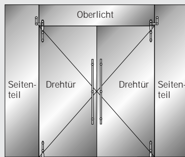
Anlagentyp 23 2 COMPACT-Sets 3 oder 9
