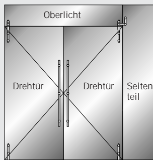
Anlagentyp 21 1 COMPACT-Set 2 oder 8 + 1 COMPACT-Set 3 oder 9
