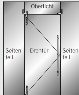
Anlagentyp 15 COMPACT-Set 3 oder 9 + 1 Oberlicht-/Seitenteilverbinder
