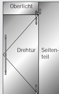
Anlagentyp 13 COMPACT-Set 3 oder 9
